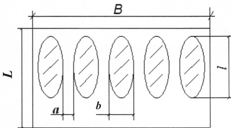
Рисунок 3 - Расположение тестовых заготовок на лотке: B - ширина лотка; L - длина лотка; a - зазор между изделиями; b - ширина изделия; l - длина изделия
