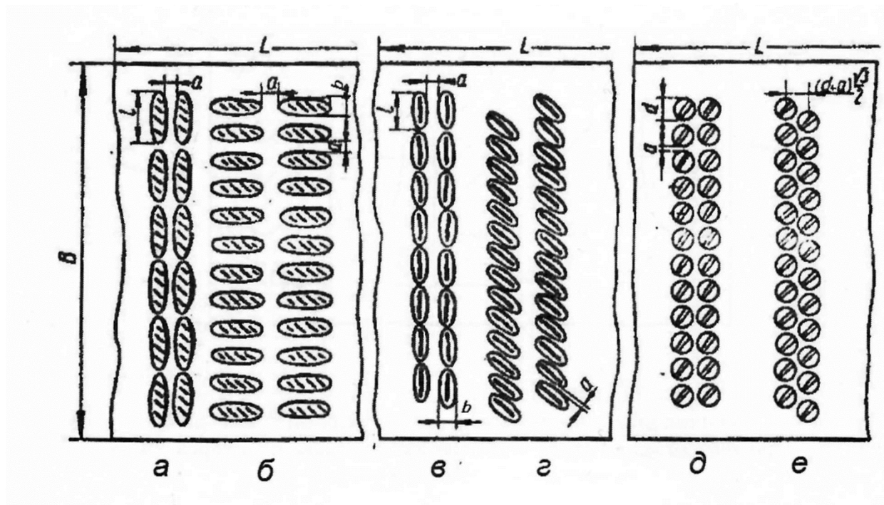
Рисунок 2 - Укладка тестовых заготовок на поду туннельной печи:
