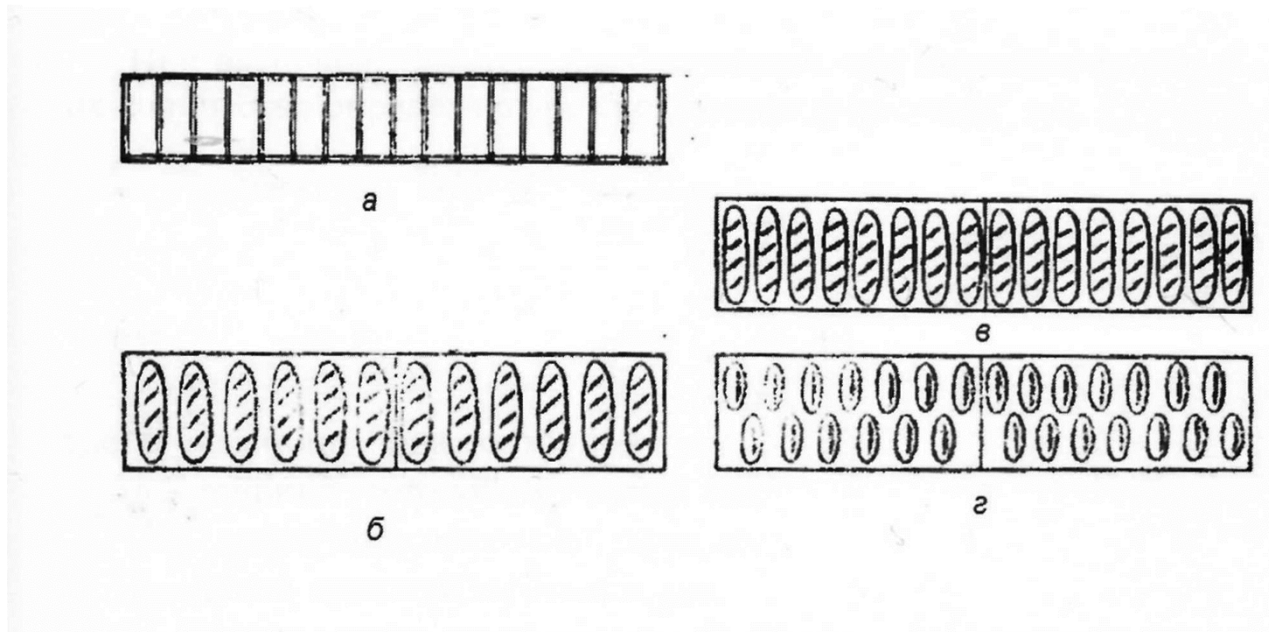
Рисунок 1 - Варианты установки форм и укладки подовых изделий на люльки тупиковых печей:
