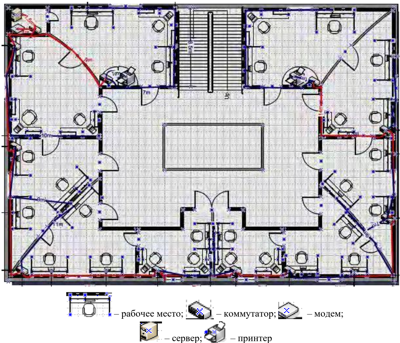
Рисунок 4 – План этажа
